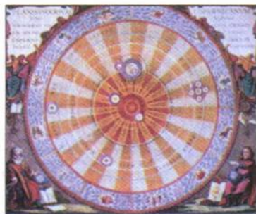
Картина мира по Копернику
